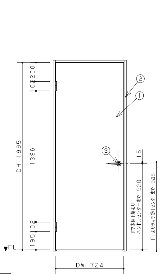
立面図
