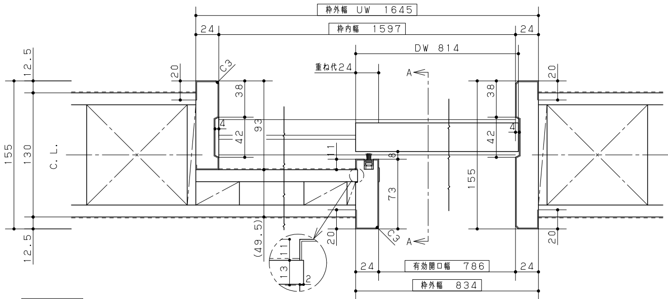
横詳細図
