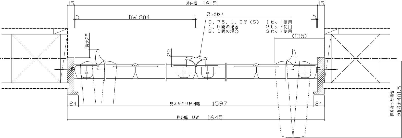
横詳細図
