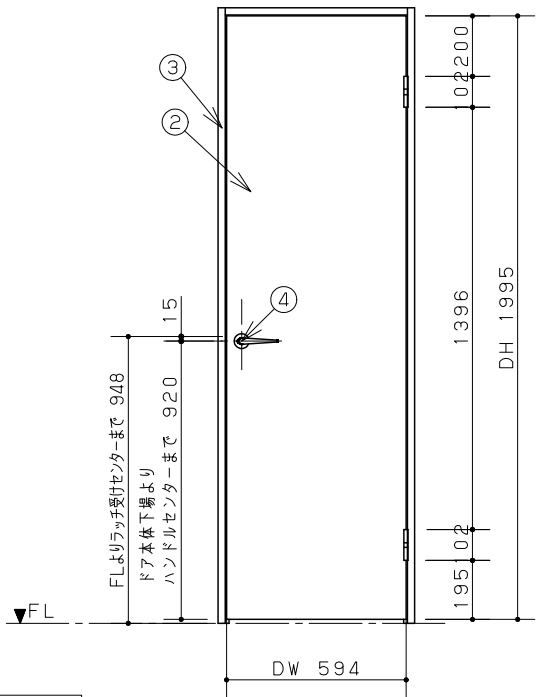
立面図
