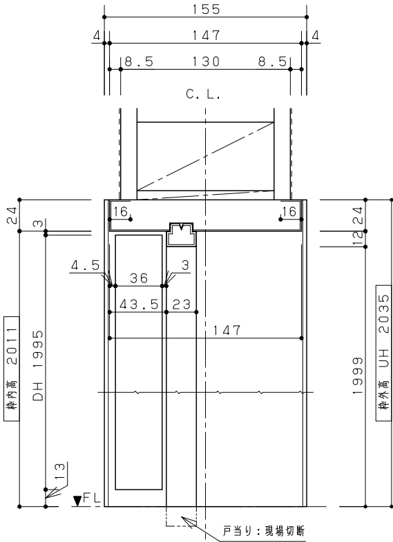
縦詳細図
