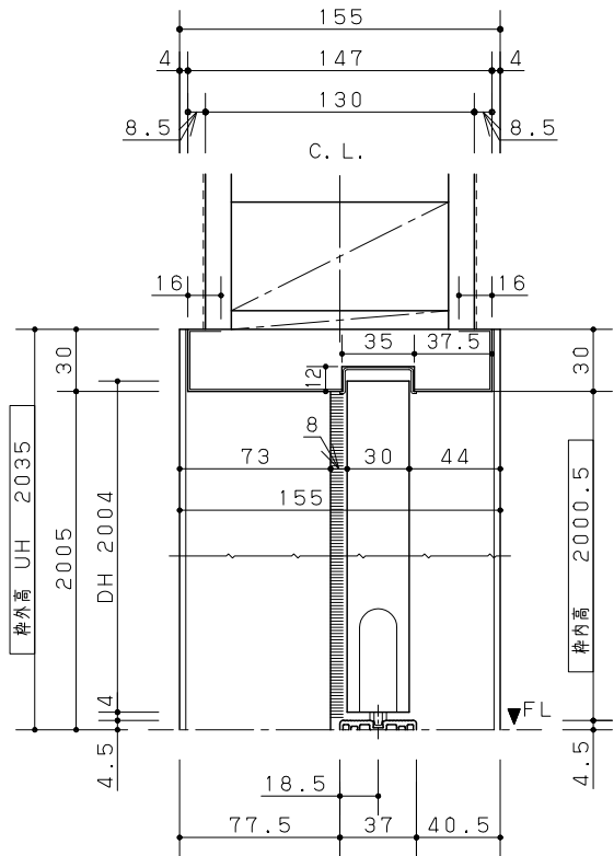
縦詳細図
