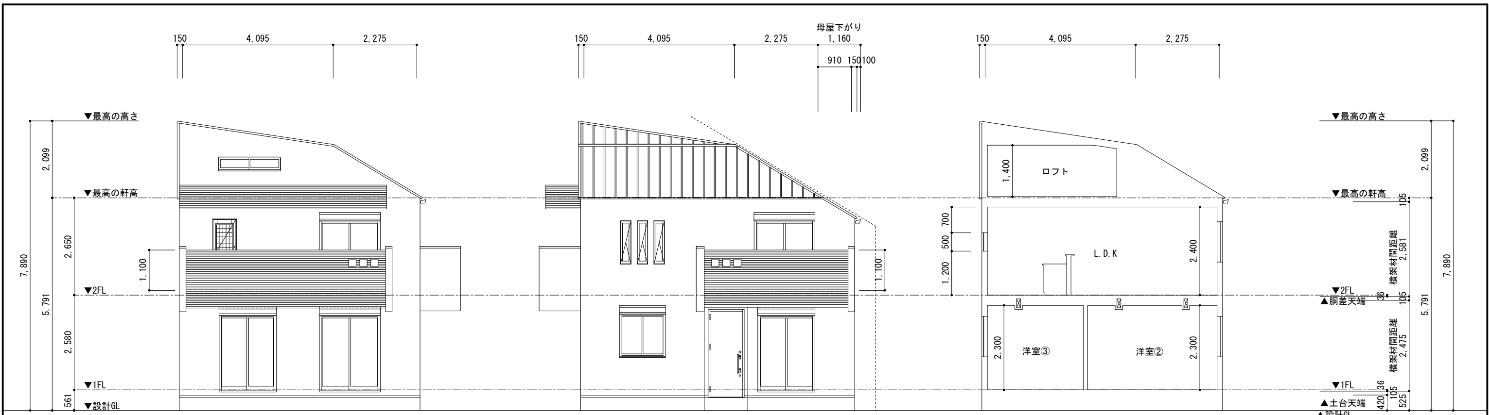
南立面図
