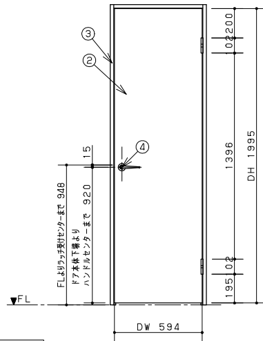
立面図
