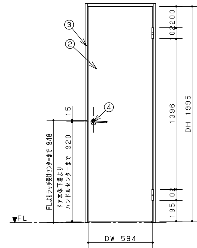
立面図
