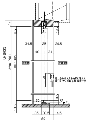
縦詳細図
