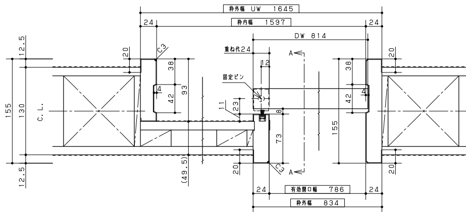
横詳細図
