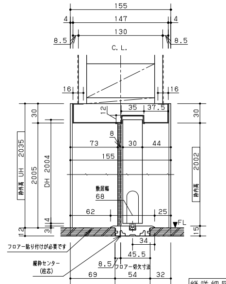
縦詳細図
