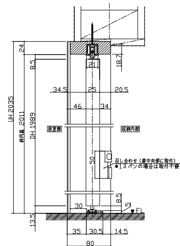
縦詳細図
