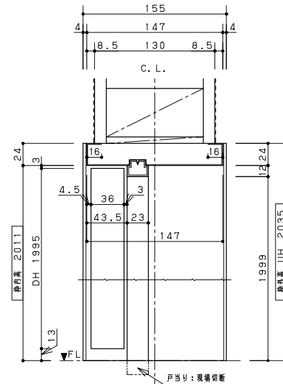
縦詳細図
