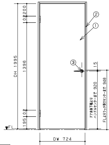
立面図
