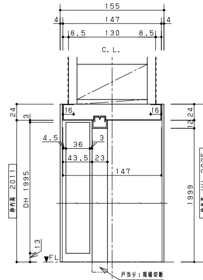
縦詳細図
