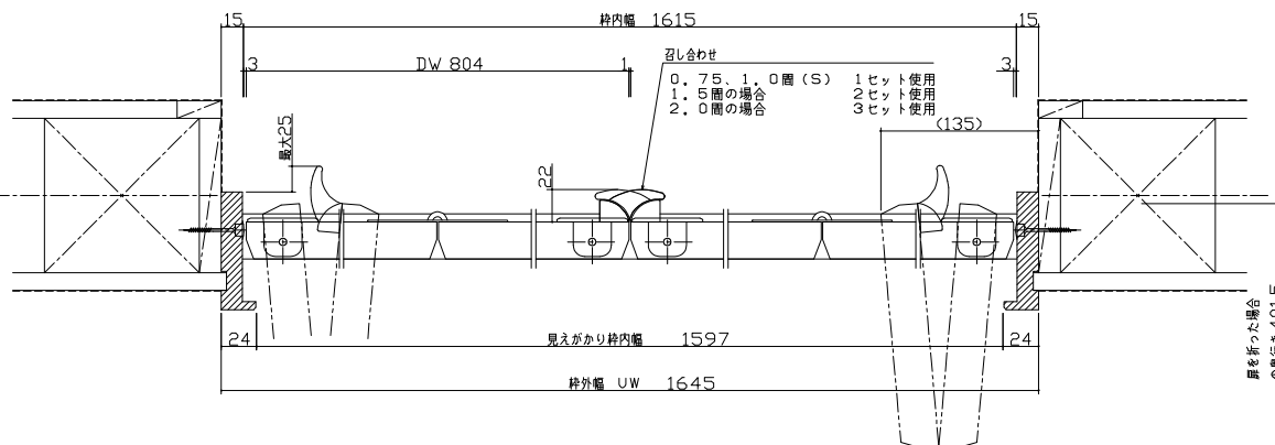
横詳細図
