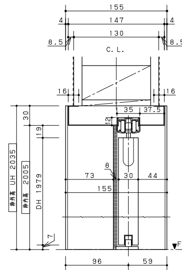
A-A断面兼透視図
