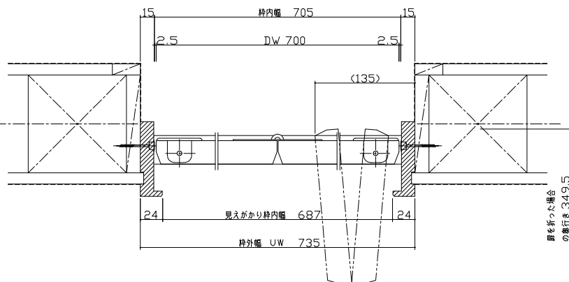
横詳細図
