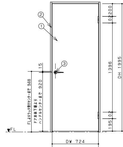
立面図
