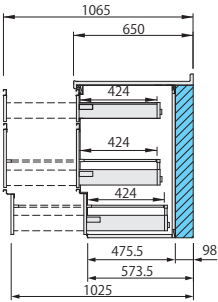
ベースキャビネット 2段引出しタイプ
