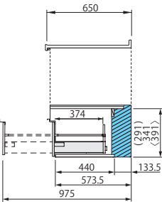
浅型食器洗い乾燥機用 キャビネット
