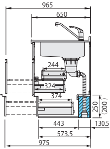
シンクキャビネット スライドボックス付
