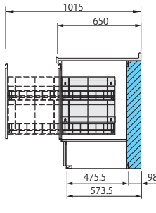
網かご付スライドキャビネット (スライド収納用)
