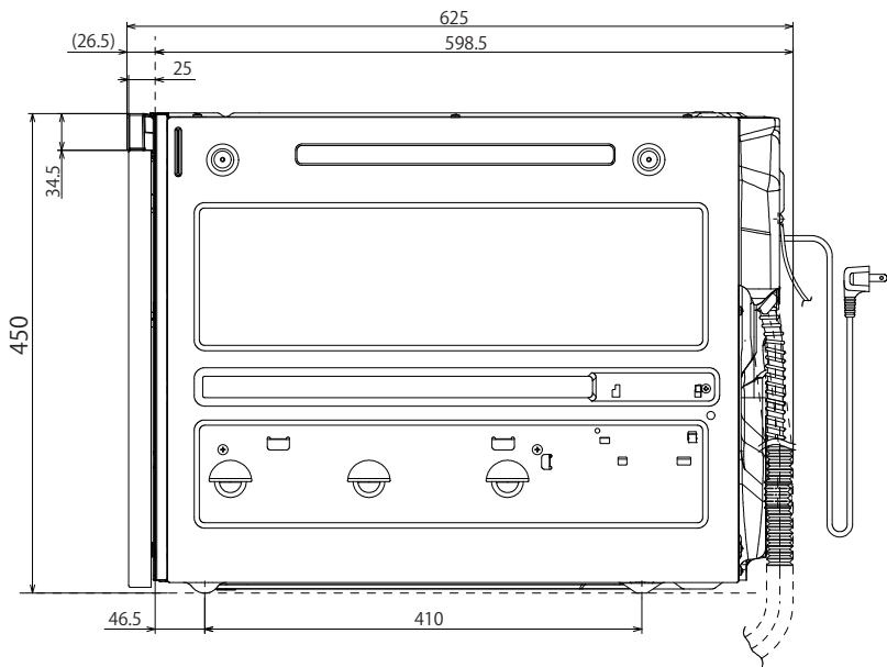
側面図
