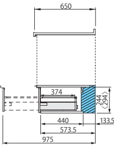
深型食器洗い乾燥機用 キャビネット
