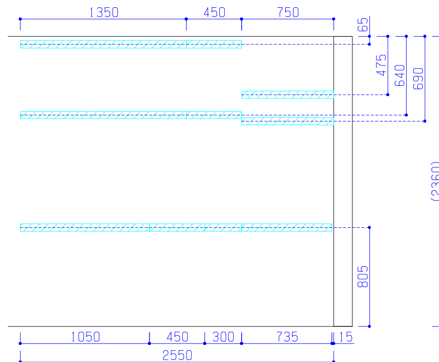
栈木展開図A
