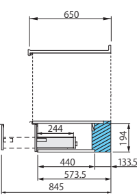
深型食器洗い乾燥機用 キャビネット (高さ80cm用)
