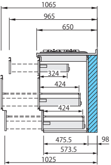
コンロキャビネット (グリルレス用)
