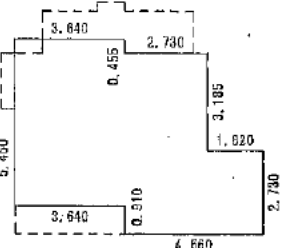
2階平面図
