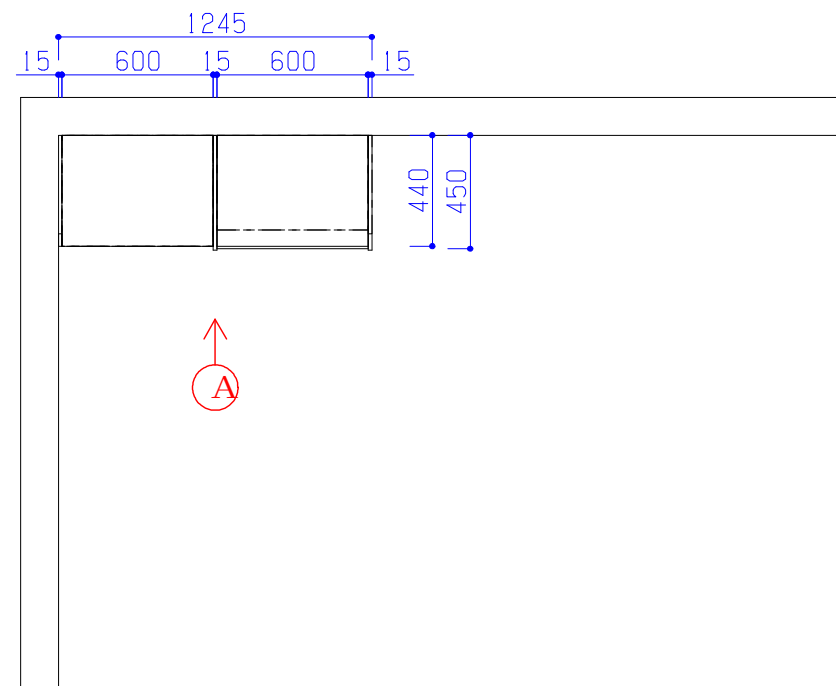
平面図
