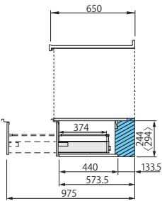
深型食器洗い乾燥機用 キャビネット
