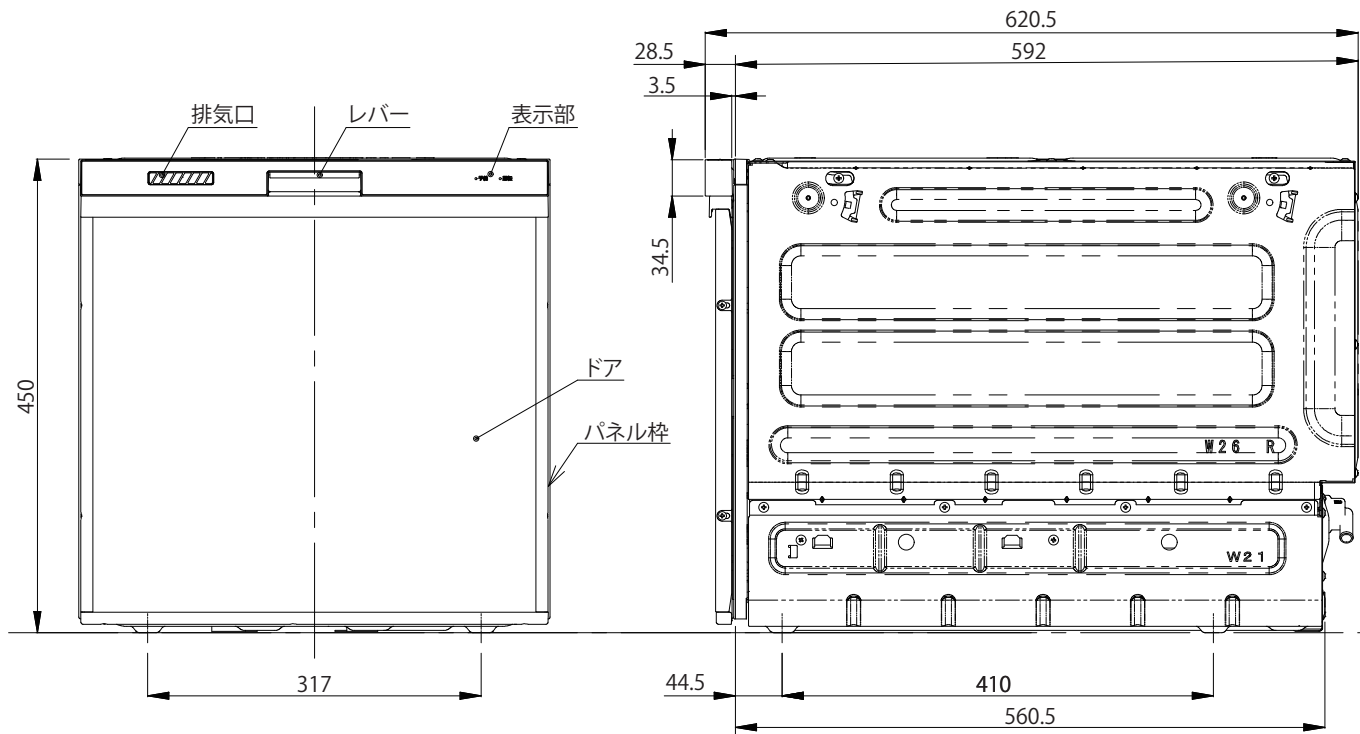
正面図
