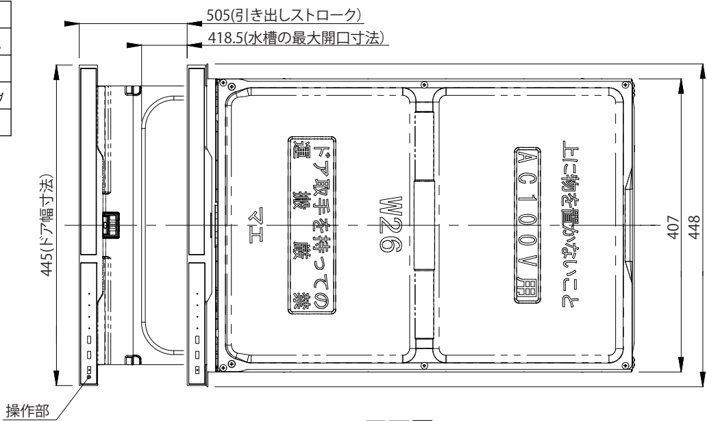
平面図
