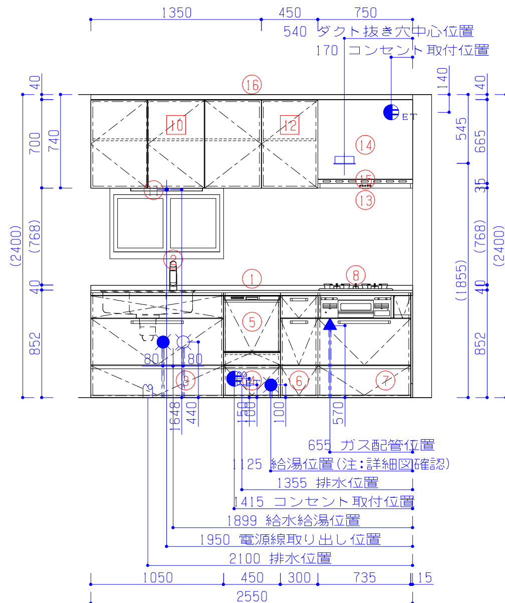
展開図A
