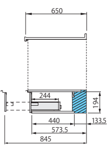
深型食器洗い乾燥機用 キャビネット (高さ80cm用)
