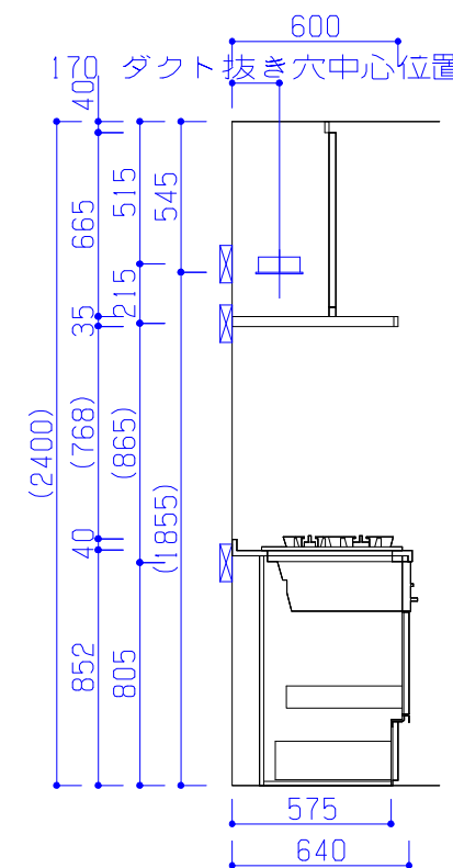
断面図B
