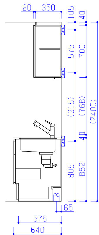
断面図A
