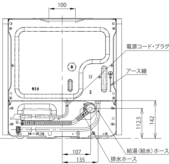
背面図
