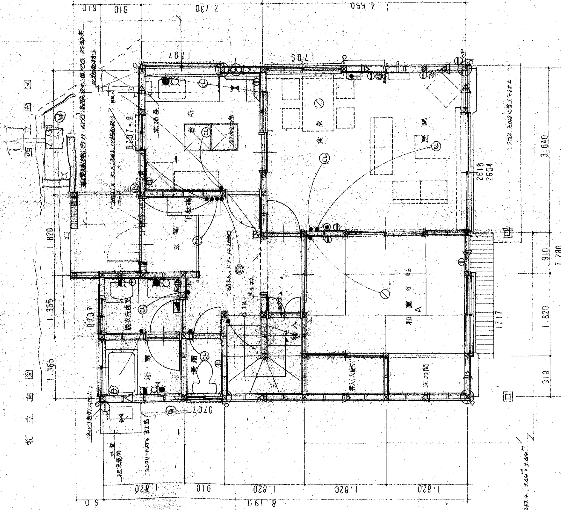
1階平面図 1/50
